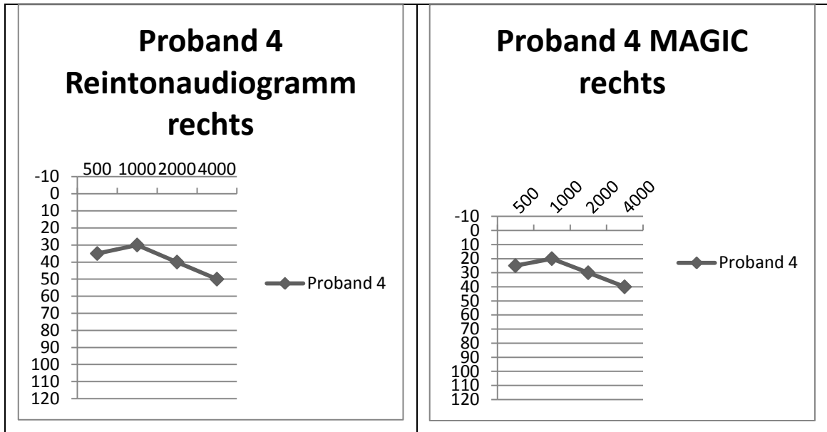
Abbildung 27: Reintonaudiogramm und MAGIC Audiogramm Proband 4 rechts
